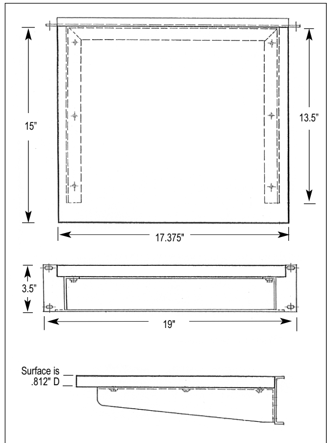
L16-3 Dimensions
